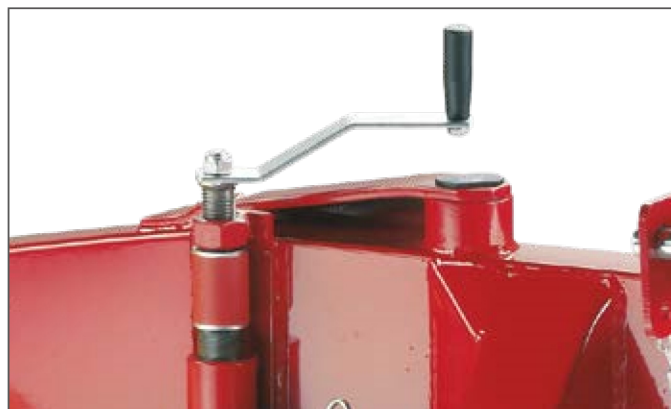
Meccanismo di scatto in caso di urti e per trasporto su strada Shutter mechanism in case of collisions and for road transport
